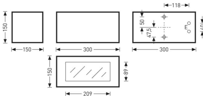
TX054493 DIN 5040: A60 UTE: 1,00 B
