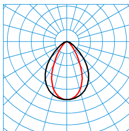
TX054493 DIN 5040: A60 UTE: 1,00 B
