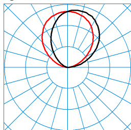
TX050885 DIN 5040: E03 UTE: 0,00 J + 1,00 T ■ C0 - C180 ■ C90 - C270
