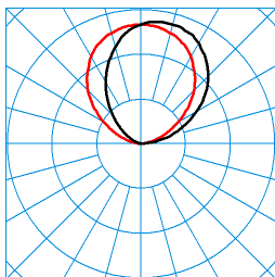
TX054684 DIN 5040: E03 UTE: 0,00 J + 1,00 T ■ C0 - C180 ■ C90 - C270
