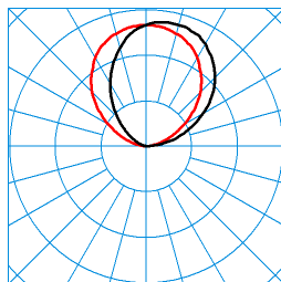
TX054685 DIN 5040: E03 UTE: 0,00 J + 1,00 T ■ C0 - C180 ■ C90 - C270
