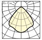
Ector M46 RMV 228--TWLi 830
