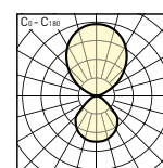
Luceo H CDP LED 6300-840... UTE: 0,38 D + 0,62 T DIN 5040: D53 CIBSE: BZ 2/2.5/BZ 3 NBN L 14-002: BZ 3
