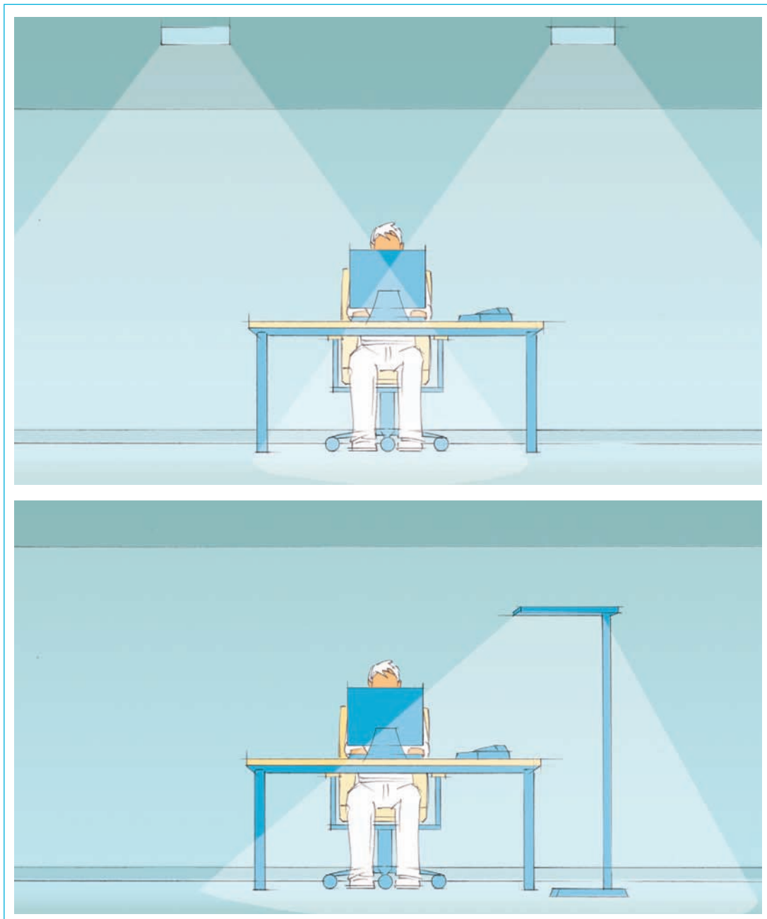
Abbildung 17 Richtiger Lichteinfall am Arbeitsplatz
