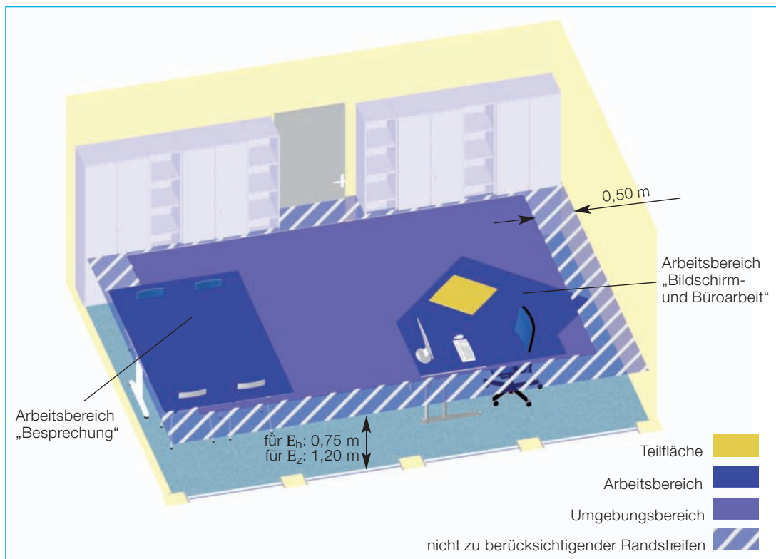
Abbildung 22 Teilflächenbezogene Beleuchtung: Bewertungsflächen für die horizontale Beleuchtungsstärke ( E_h ) und die zylindrische Beleuchtungsstärke ( E_z )
