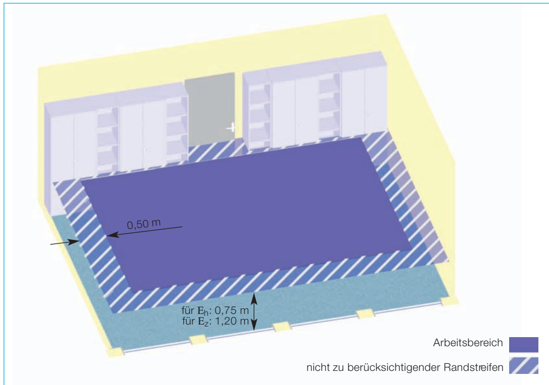
Abbildung 19 Raumbezogene Beleuchtung: Bewertungsflächen für die horizontale Beleuchtungsstärke ( E_h ) und die zylindrische Beleuchtungsstärke ( E_z )
