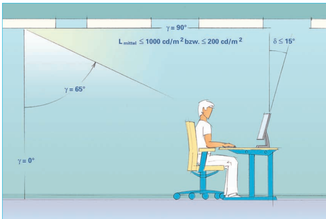
Abbildung 11 Kritischer Bereich ( \gamma \geq 65^\circ ) für Leuchtdichten von Leuchten, die zu Reflexblendung auf dem Bildschirm führen können
