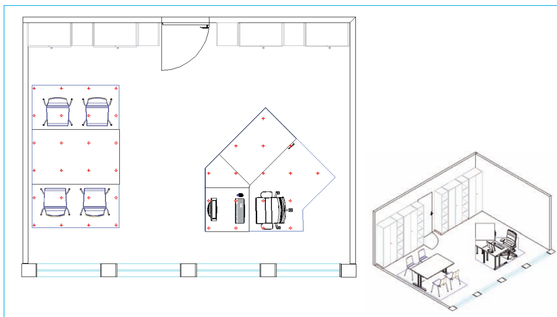
Abbildung 5 Beispiel für die Verteilung von Messpunkten für die mittlere horizontale Beleuchtungsstärke in zwei Arbeitsbereichen (Rastermaß 0,5 m)
