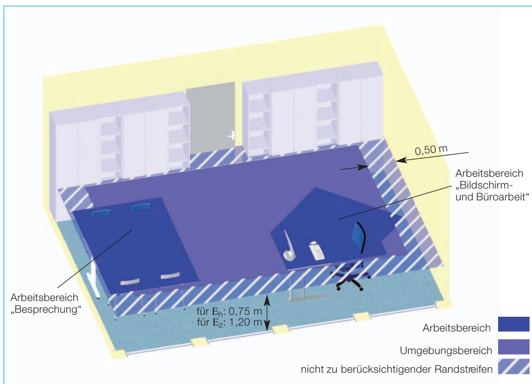
Abbildung 21 Arbeitsbereichsbezogene Beleuchtung: Bewertungsflächen für die horizontale Beleuchtungsstärke ( E_h ) und die zylindrische Beleuchtungsstärke ( E_z )
