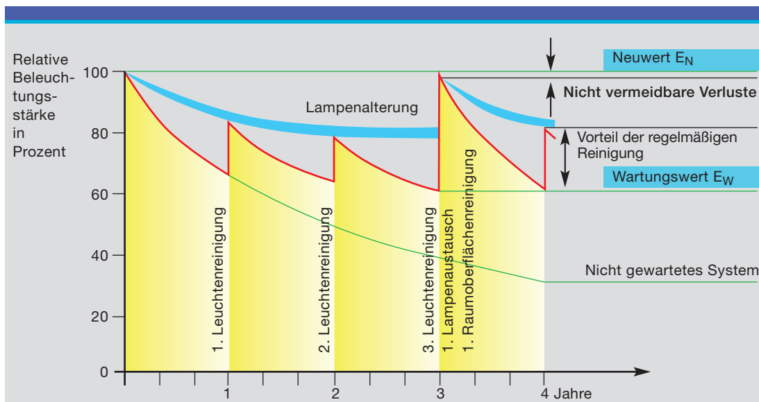
Abbildung 28 Zusammenhang zwischen dem Absinken der Beleuchtungsstärke und der Wartung der Beleuchtungsanlage
