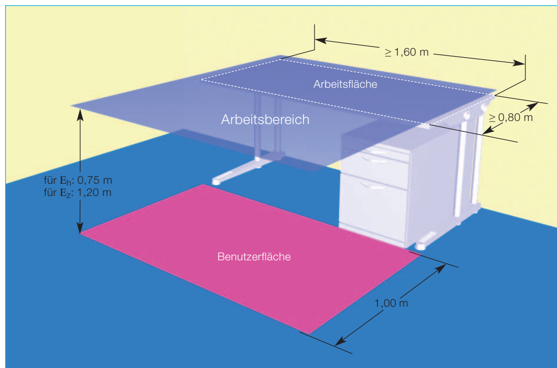
Abbildung 20 Bewertungsfläche für die horizontale Beleuchtungsstärke ( E_h ) und zylindrische Beleuchtungsstärke ( E_z ) im Arbeitsbereich
