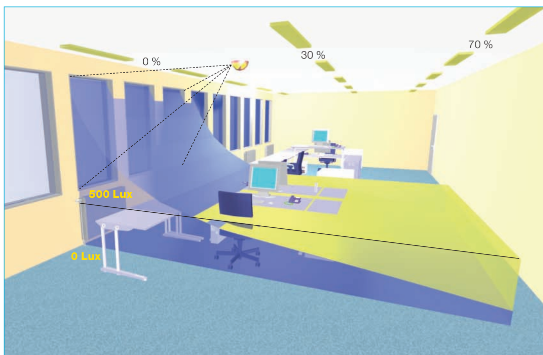
Abbildung 26 Steuerung der Beleuchtungsanlage (siehe Prozentangaben) in Abhängigkeit des einfallenden Tageslichts
