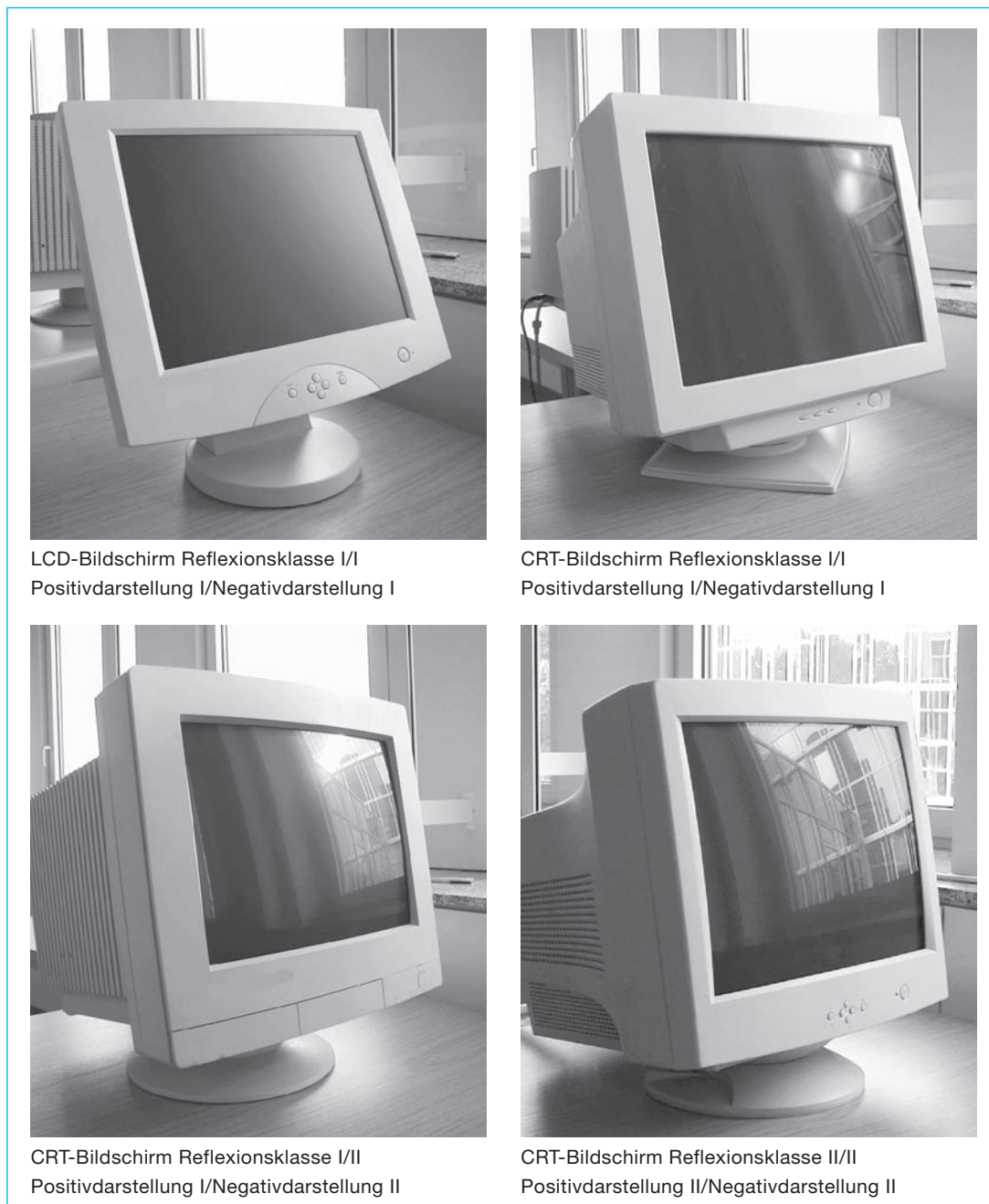
Abbildung 7 Spiegelbilder auf Bildschirmen verschiedener Reflexionsklassen
